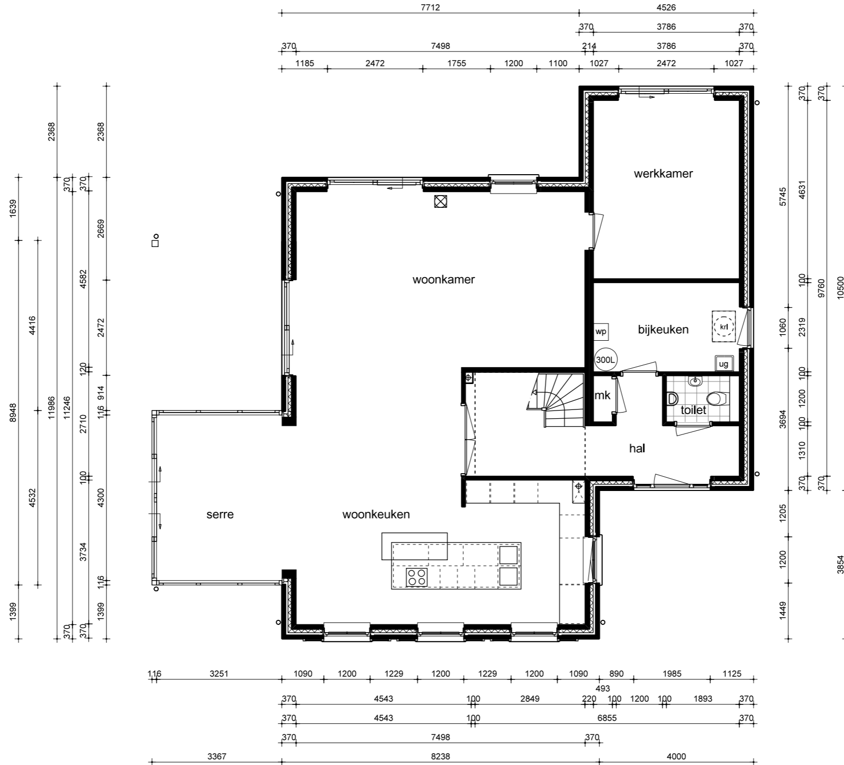
begane grond
