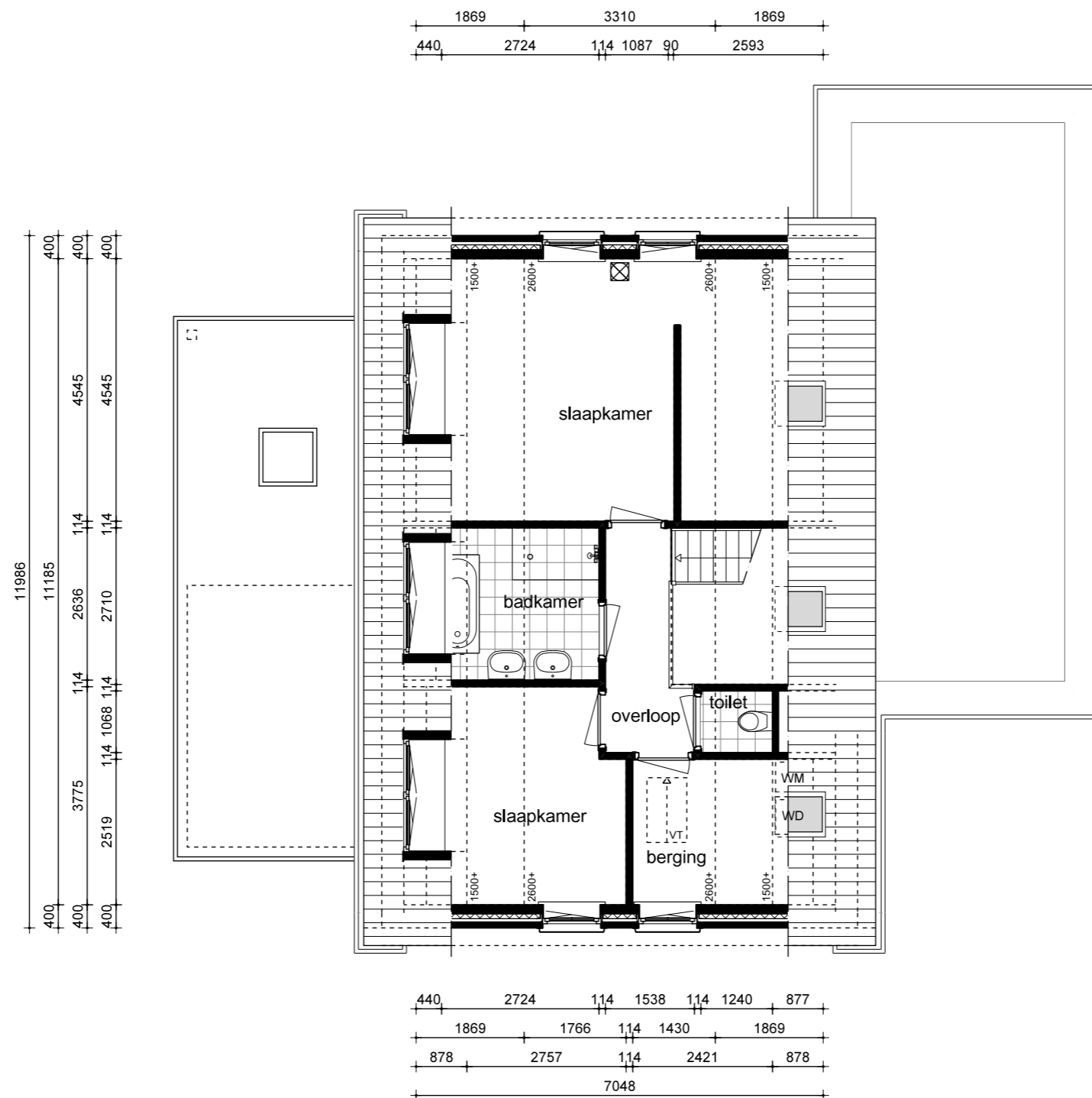
1e verdieping
