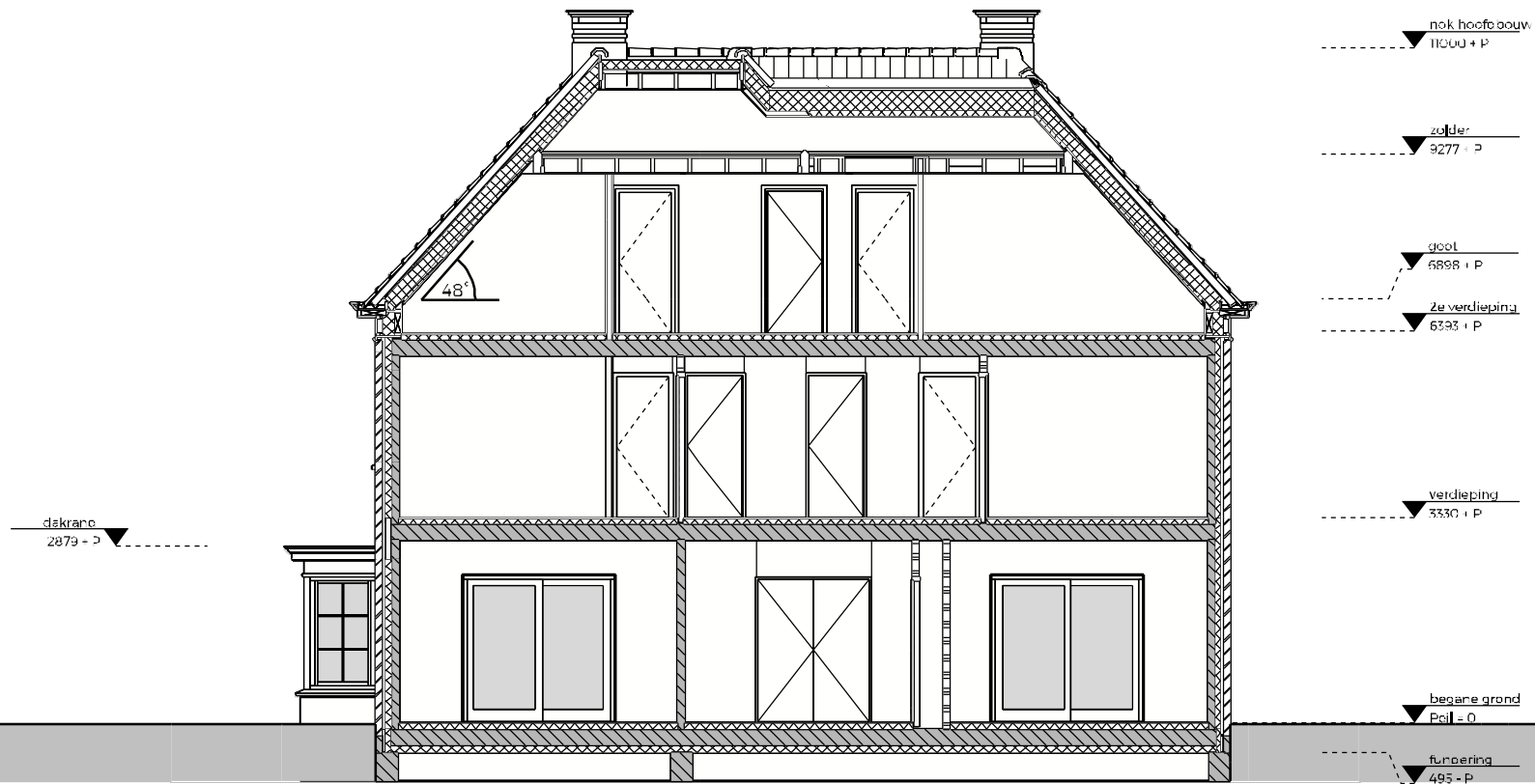
doorsnede A-A
