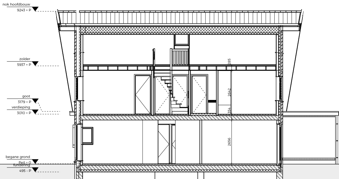
Doorsnede B-B
