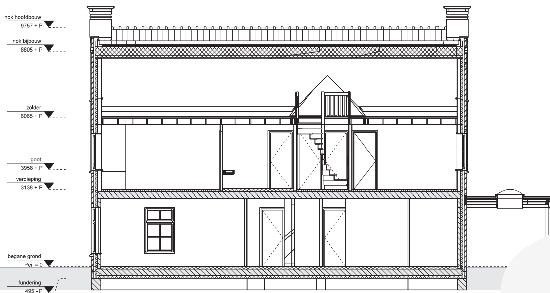
Doorsnede B-B
