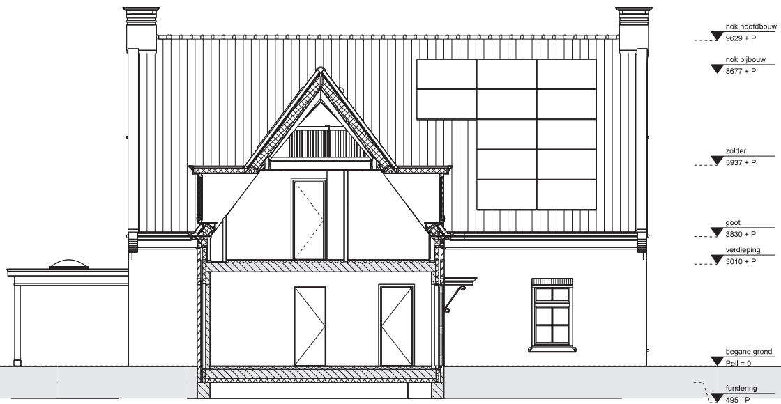
Doorsnede C-C
