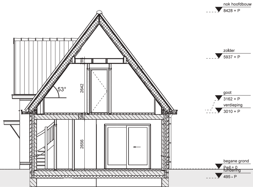
Doorsnede A-A
