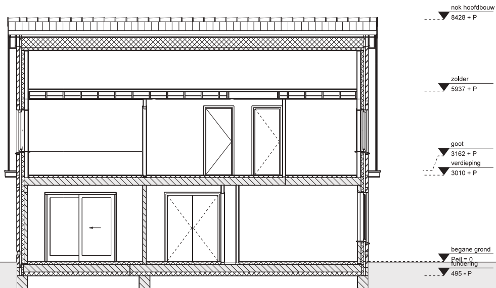
Doorsnede B-B
