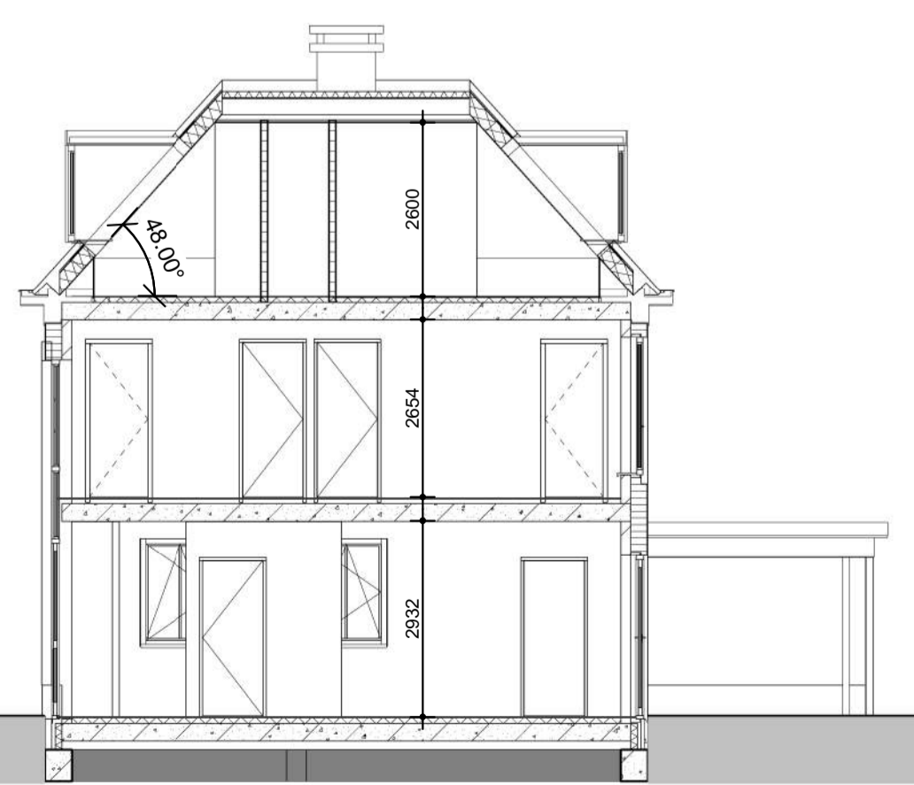
doorsnede A-A
