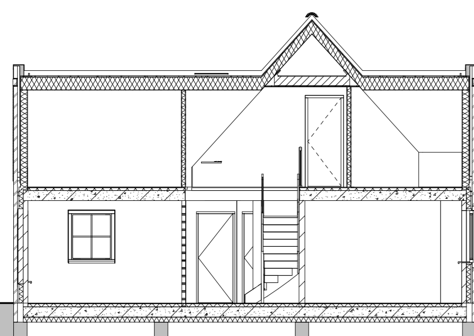
Doorsnede A-A
