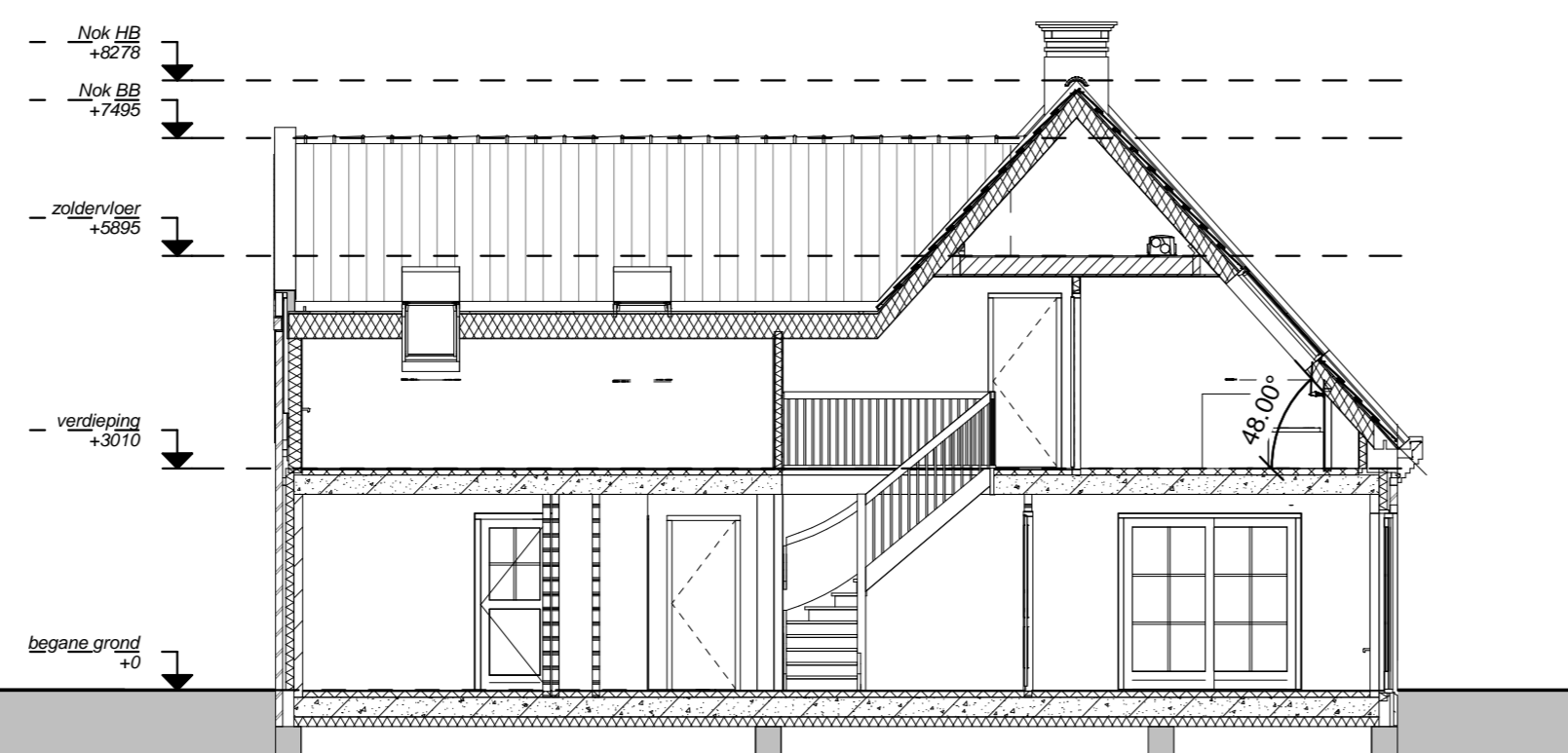
Doorsnede B-B
