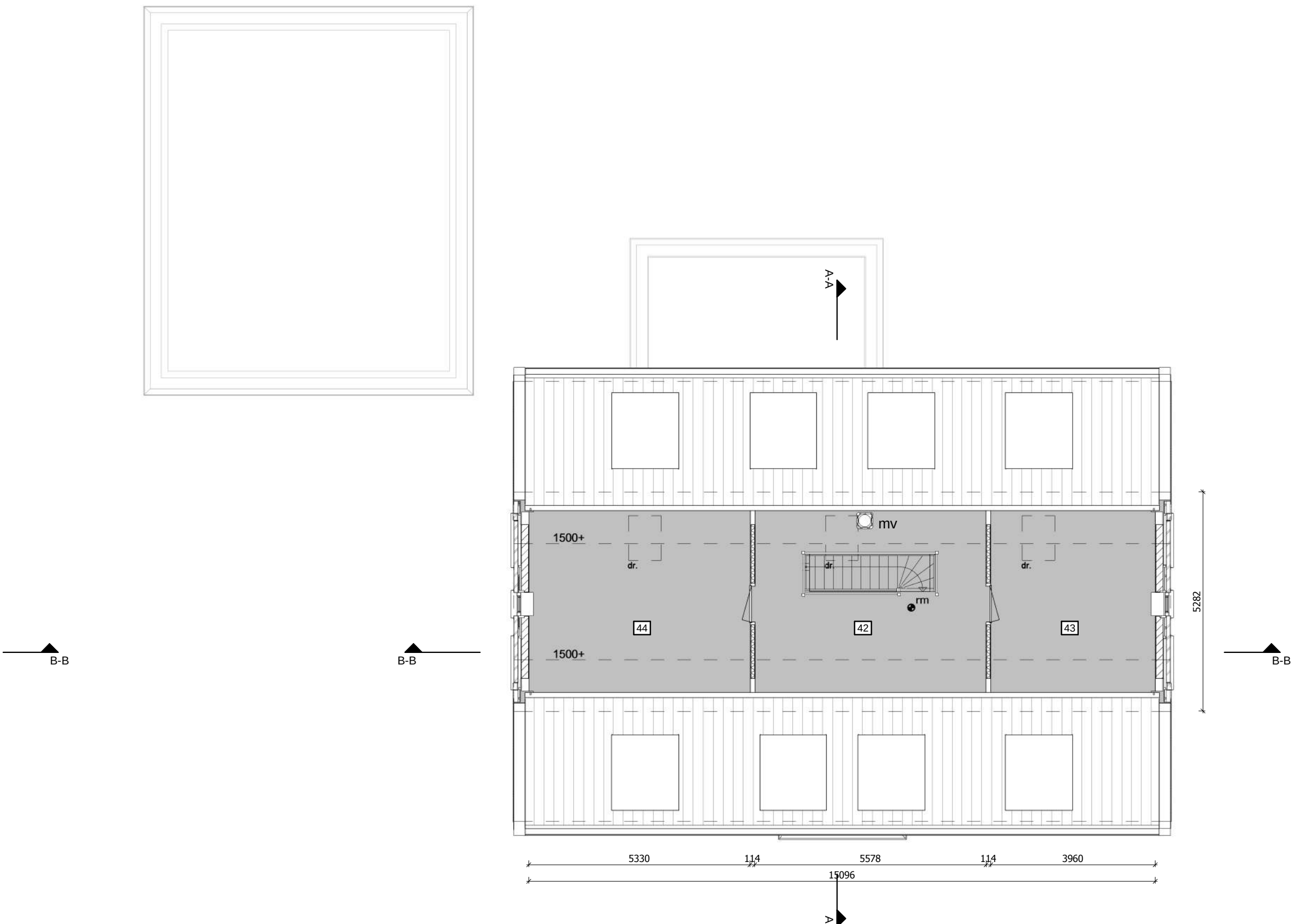
zoldervloer
