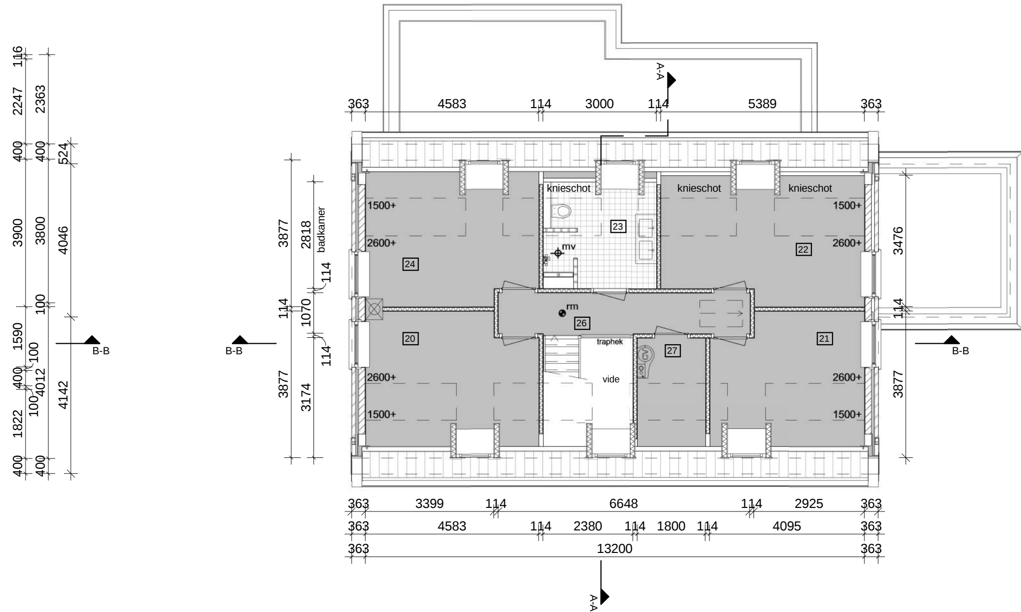
verdieping
