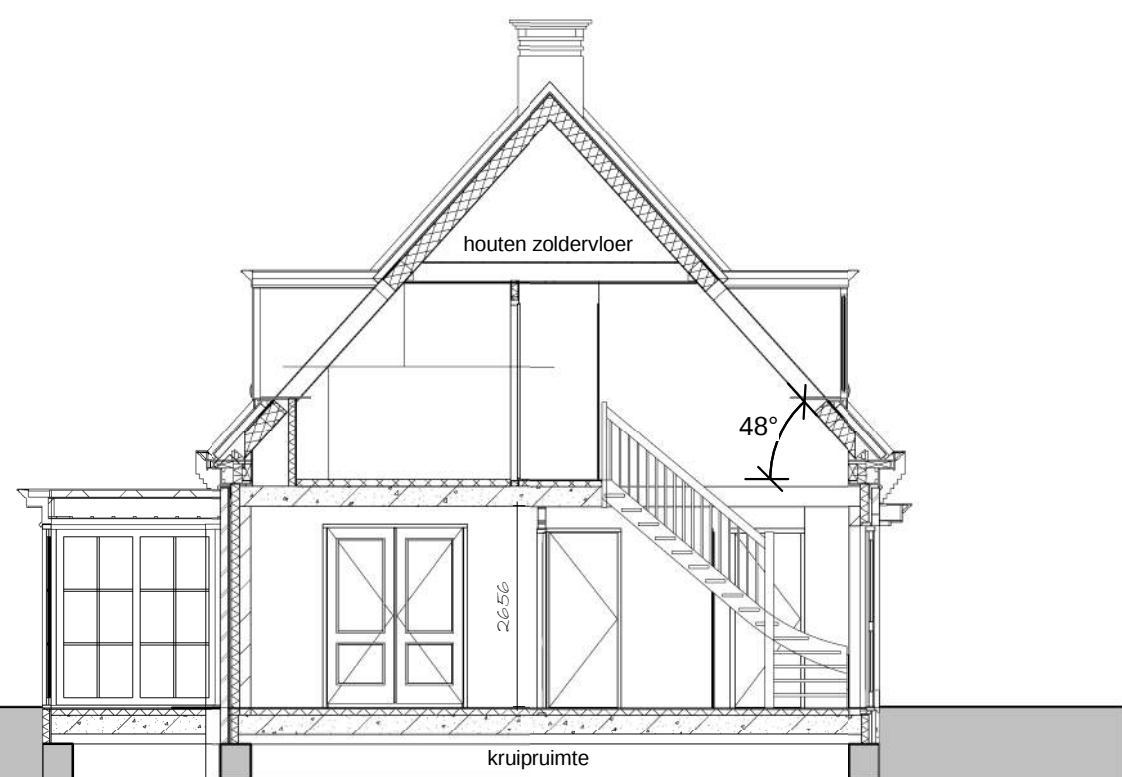
doorsnede A-A
