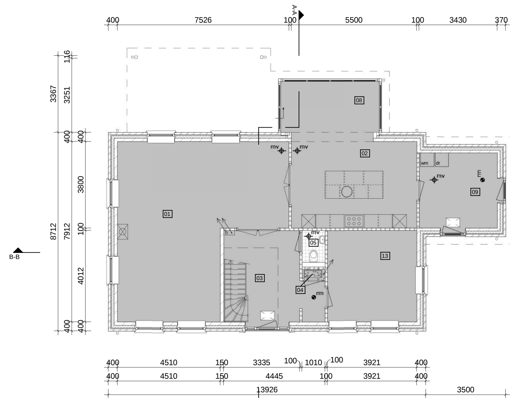
begane grond
