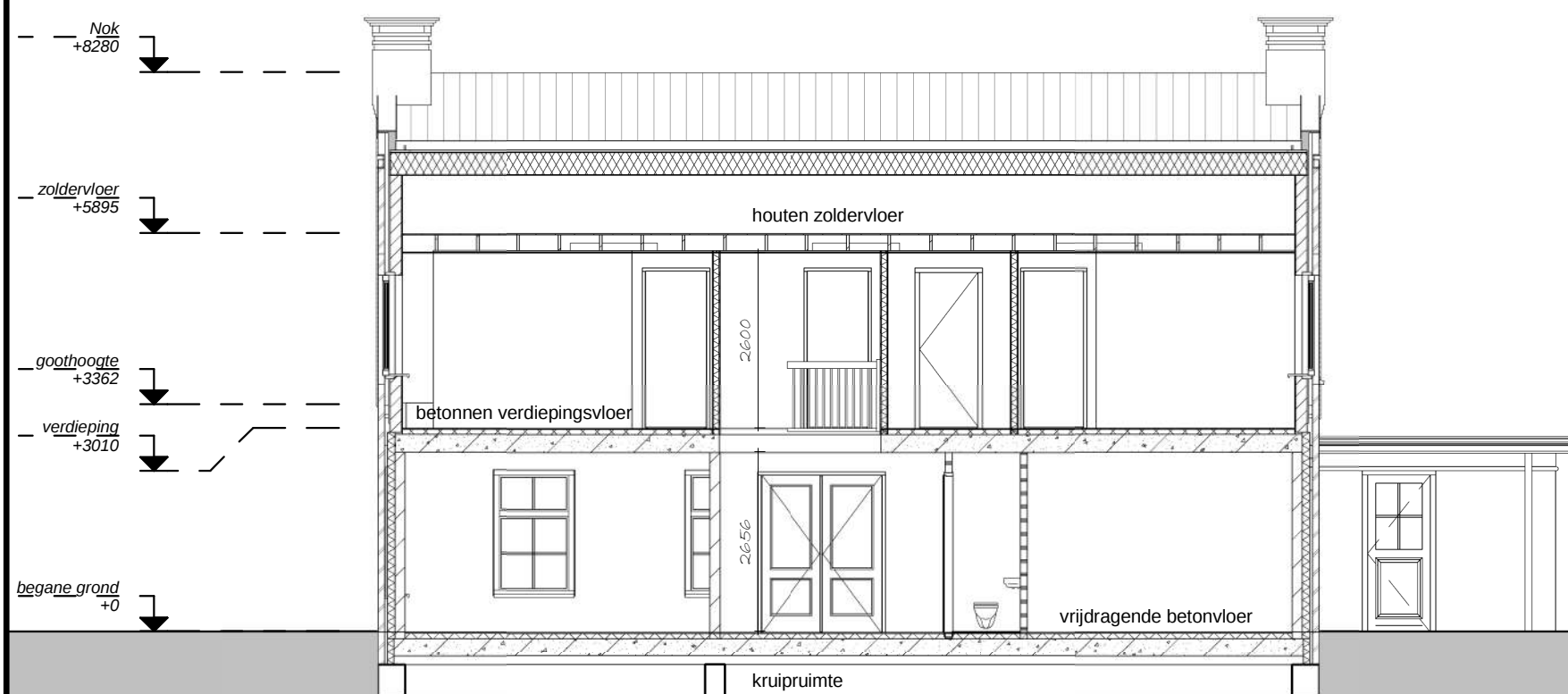
doorsnede B-B
